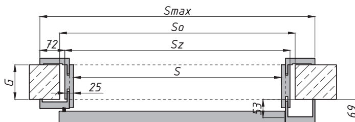
Drzwi przesuwane na ścianę Pojedyncze
