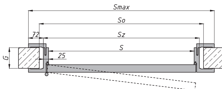
Drzwi jednoskrzydłowe
