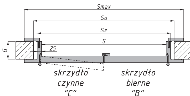
Drzwi dwuskrzydłowe
