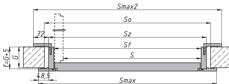
Drzwi REWERSYJNE jednoskrzydłowe
