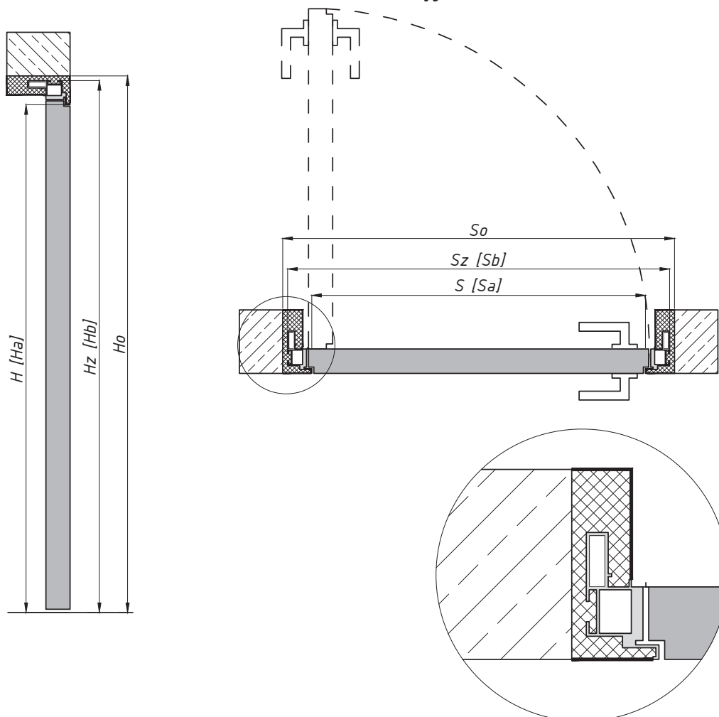
Drzwi z ościeżnicą aluminiową otwierane rewersyjnie
